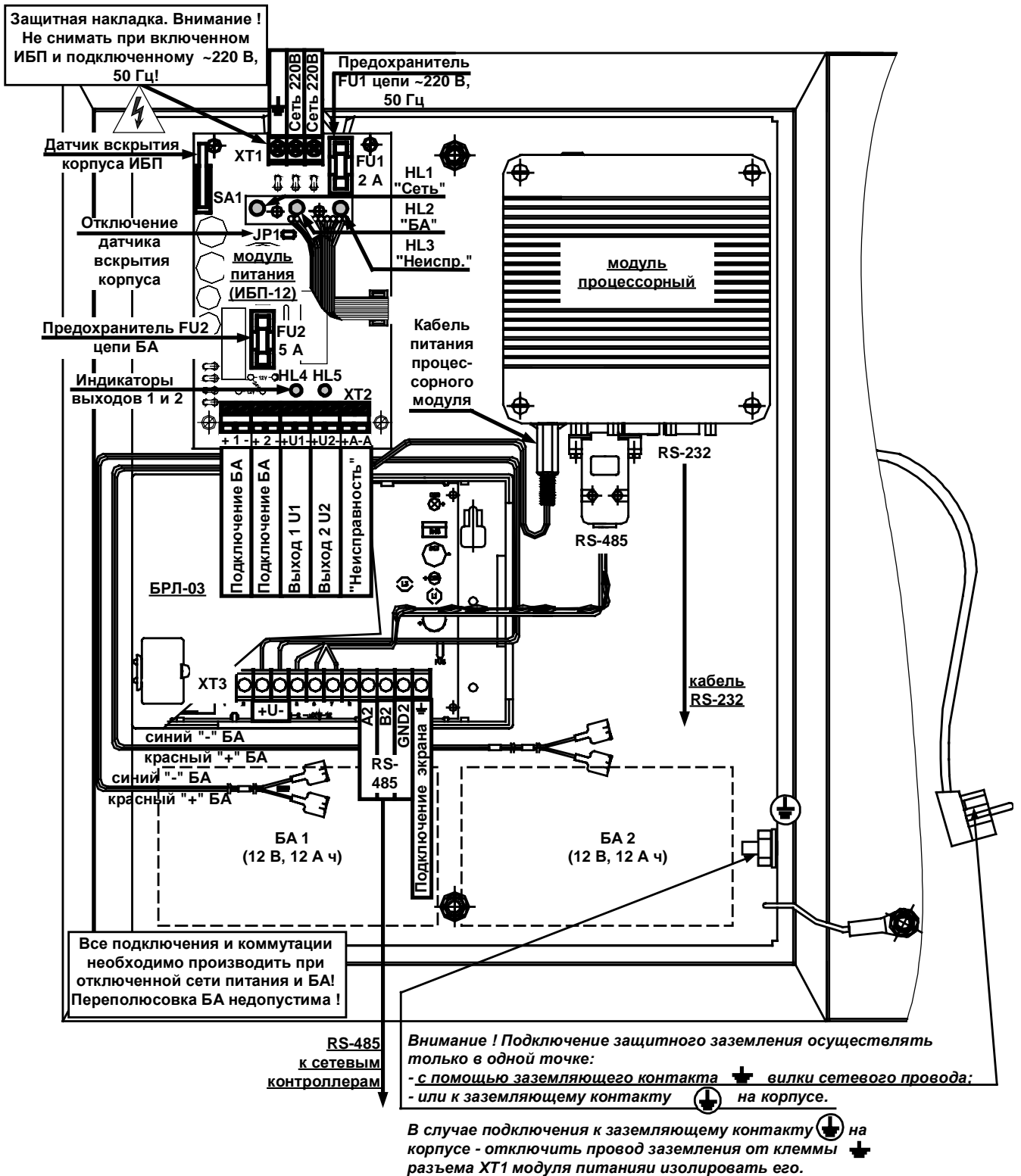
Рис. 4 БЦП, расположение элементов, подключение.
