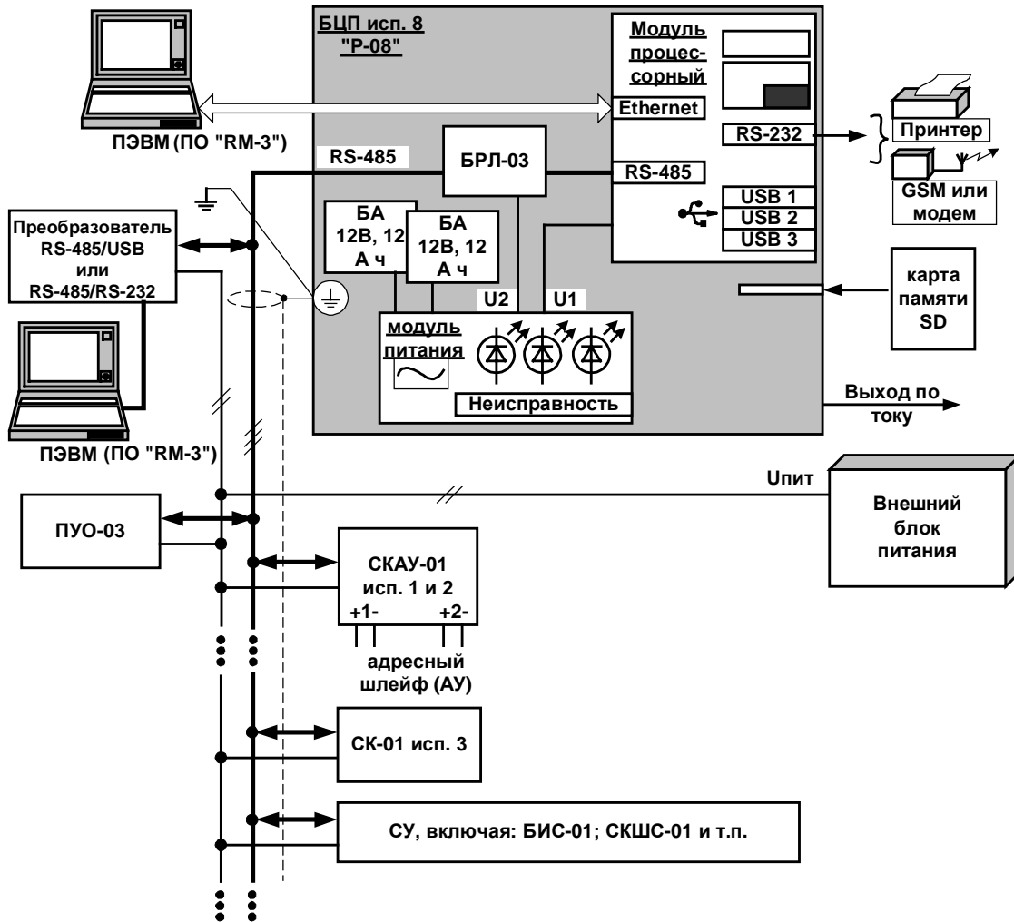
Рис. 2 Использование (подключение) БЦП исп. 8. Структурная схема БЦП.
