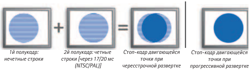
РИС 3.5а Слева показано как выглядит чересстрочное изображение на экране с прогрессивной разверткой (компьютерном мониторе). Справа показано как выглядит изображение с прогрессивной разверткой на компьютерном мониторе.
