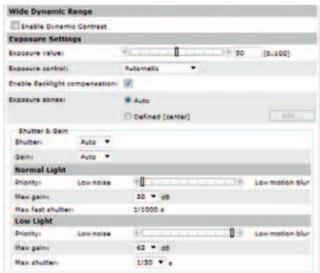
Рис 3.6а Страницка с параметрами настройки видеокамеры, среди которых есть параметры для условий низкой освещенности.
