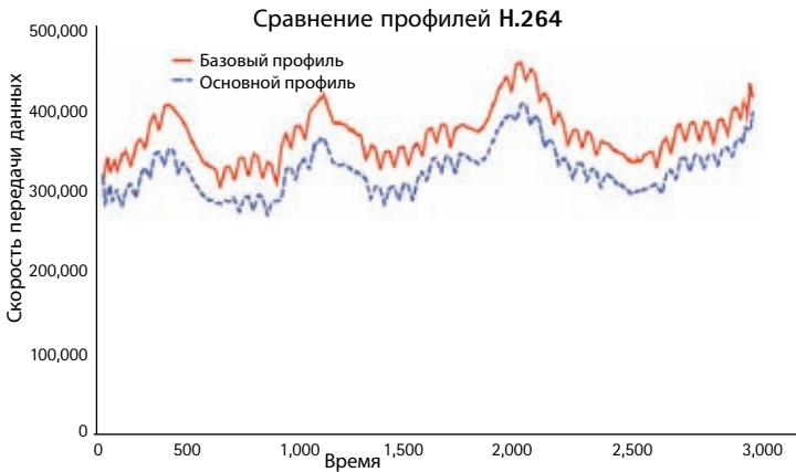
РИС 7.2а При сопоставимом качестве изображения, видеокодек Main Profile H.264, используемый компанией Axis, даёт меньший битрейт, чем видеокодек Baseline Profile H.264.
