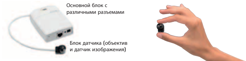
РИС 2.4ф Малоаметная сетевая видеокамера, например показанная выше модель AXIS P12, органично вписывается в любой интерьер. Оптический блок можно установить практически в любом месте: за тонким листом металла дверного проема, в любой стенке, в банкомате или отдельно в специальном корпусе. Блок электроники устанавливается отдельно от оптического блока на расстоянии до 8 метров (26 футов).
