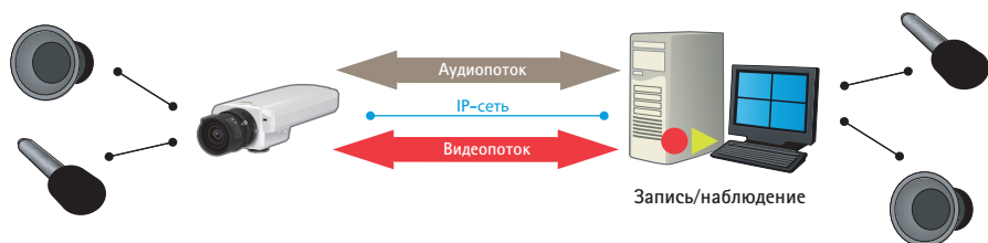
РИС 8.2а Система сетевого видеонаблюдения со встроенной поддержкой звука. Видео и аудио потоки передаются по одному сетевому кабелю.
