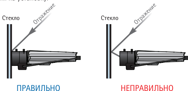
РИС 5.4а При установке видеокамеры в кожух следите, чтобы объектив вплотную прилегал к поверхности стекла, чтобы не было отражений.
