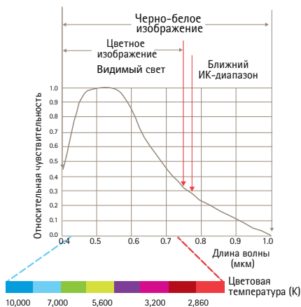
РИС 3.3b На графике показано как матрица улавливает видимый свет и излучение ближней области инфракрасного спектра с длиной волны от 0,7 мкм до 1,0 мкм.
