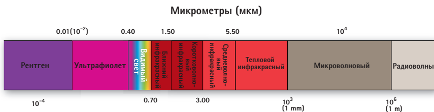
РИС 2.4n Обычные видеокамеры работают в диапазоне видимого света, т.е. где длина волны примерно от 0,4 до 0,7 мкм. Тепловизионные камеры способны улавливать излучение в гораздо более широком инфракрасном спектре, примерно до 14 мкм (шаг спектральных диапазонов указан выше не в масштабе).
