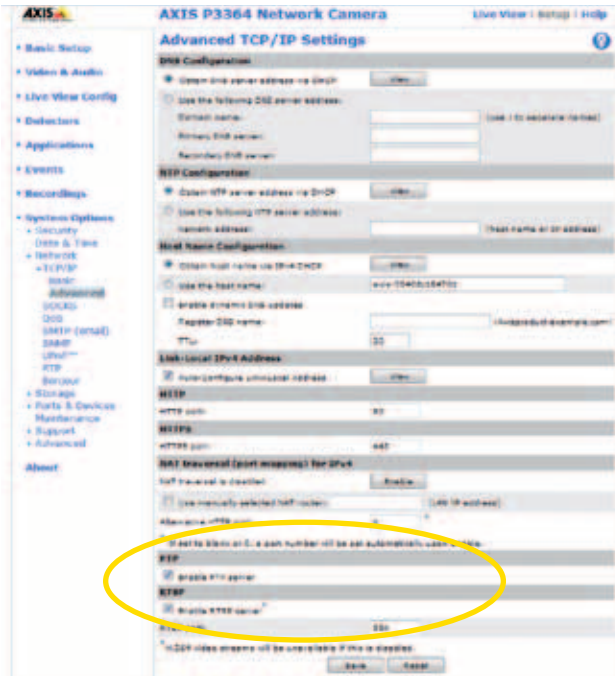
РИС 9.2b Сетевая видеоаппаратура Axis поддерживает функцию NAT traversal для настройки переадресации портов.
