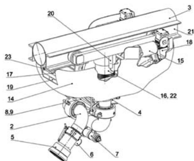
Рис. 9.8. Пожарный робот на болиде. Общий вид.
