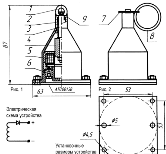
Рис. 6.1. Устройства УСП 101-72 и УСП 101-Р.
