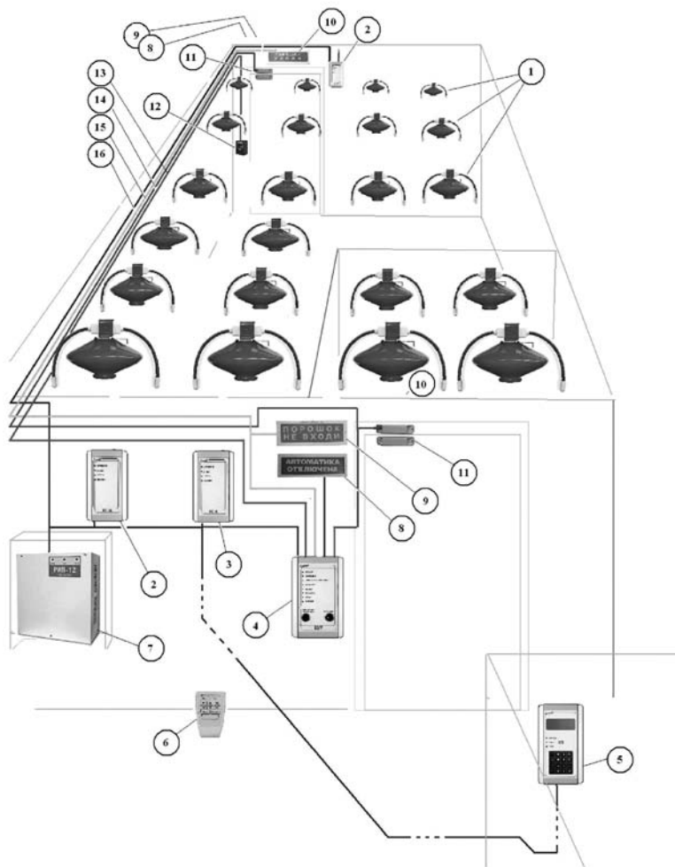
Рис. 5.5. Беспроводная система модульного пожаротушения АУП «Гарант-Р». Цифрами на рисунке обозначены: 1 – МПП с БОС; 2 – РС-М; 3 – РС-К; 4 – БУР; 5 – КП; 6 – БД; 7 – РИП; 8 – Табло «Автоматика отключена»; 9 – Табло «Порошок. Не входи!» (снаружи); 10 – Табло «Порошок. Уходи!» (внутри); 11 – Датчик контроля двери; 12 – Ручной ПИ; 13 – ШС ручных ПИ; 14 – ШС датчика контроля двери; 15 – линия управления табло; 16 – линия питания 12 вольт.
