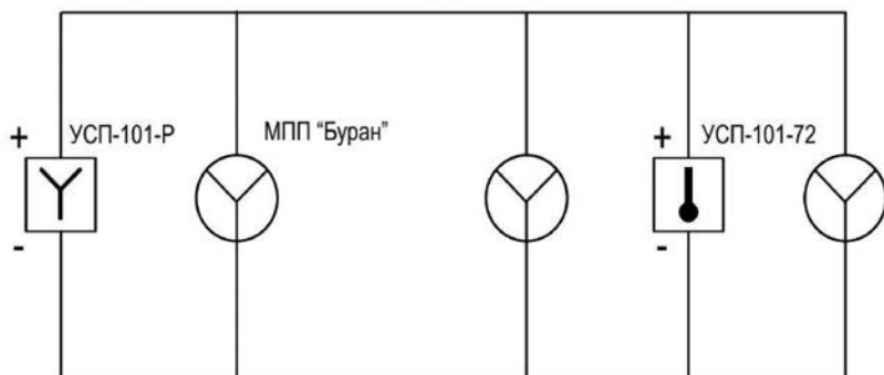
Рис. 6.4. Вариант применения устройства автоматического УСП-101 и ручного УСП-101Р.
