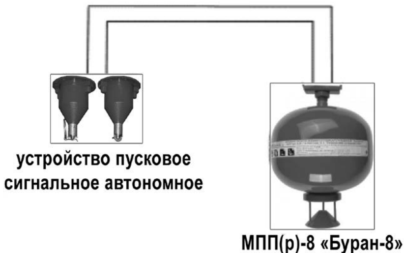
Рис. 6.5. Вариант применения УСП-101 с минимальной инерционностью срабатывания установки.
