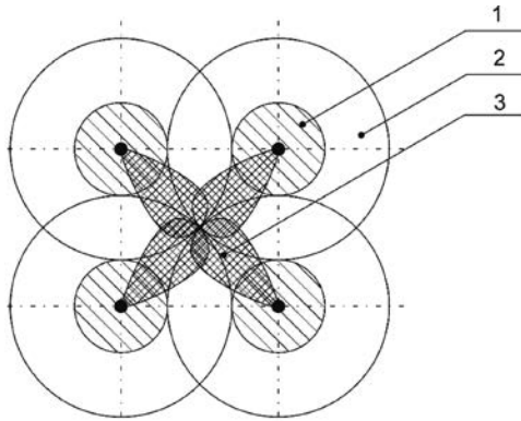
Рис. 9.4. Схема распыления при роботизированном управлении подачей огнетушащего вещества. 1 – Потенциально защищаемая площадь согласно рис. 9.3 без управлением подачи огнетушащего вещества; 2 – Потенциально защищаемая площадь при условии роботизированного управления подачи огнетушащего вещества; 3 – Реально защищаемая площадь при возникновении загорания а наиболее удаленной точке.
