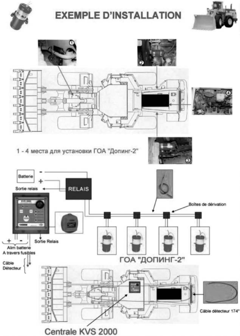
Рис. 7.5. Пример защиты тяжелой дорожной и строительной техники.
