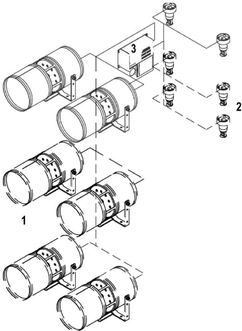
Рис. 2.3. Автономная установка пожаротушения на базе генераторов огнетушащего аэрозоля АГС-7 (1), автономных тепловых пусковых элементов ТПЭ (2) и автономной кнопки ручного пуска (3).
