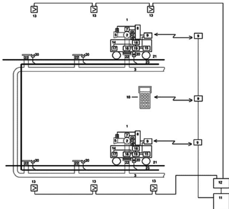
Рис. 9.7. Функциональная схема АУП РПК.
