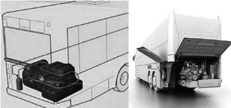
Рис. 7.23. Принципиальная схема размещения АСП-02 в моторном отсеке автобуса с задней компоновкой двигателя.
