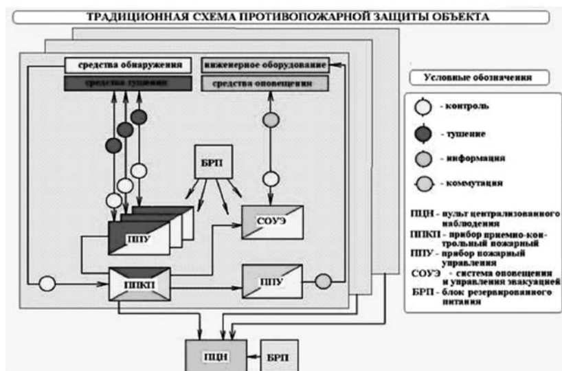
Рис. 5.1. Традиционная система управления автоматическими установками пожаротушения.
