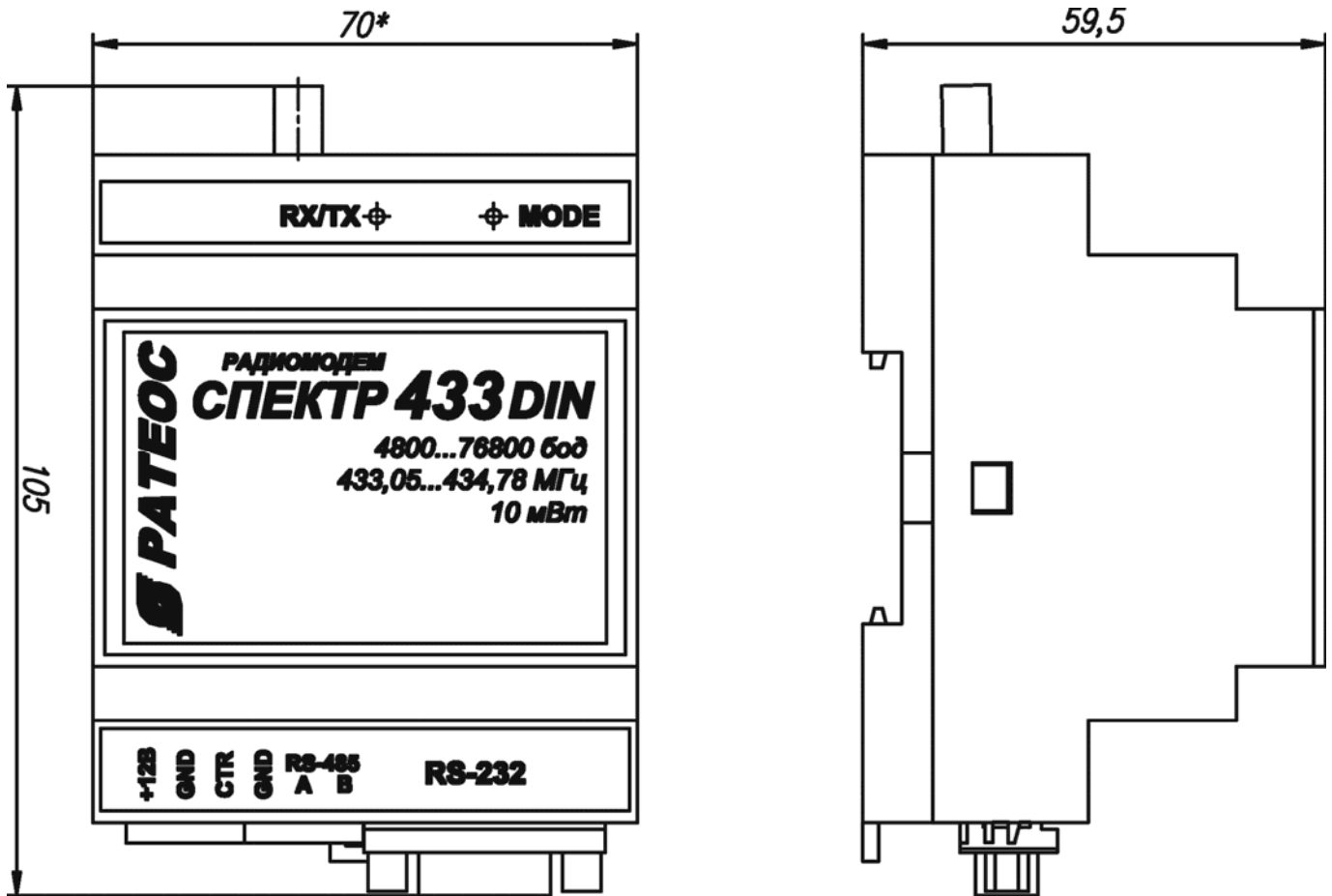
Исполнение DIN
