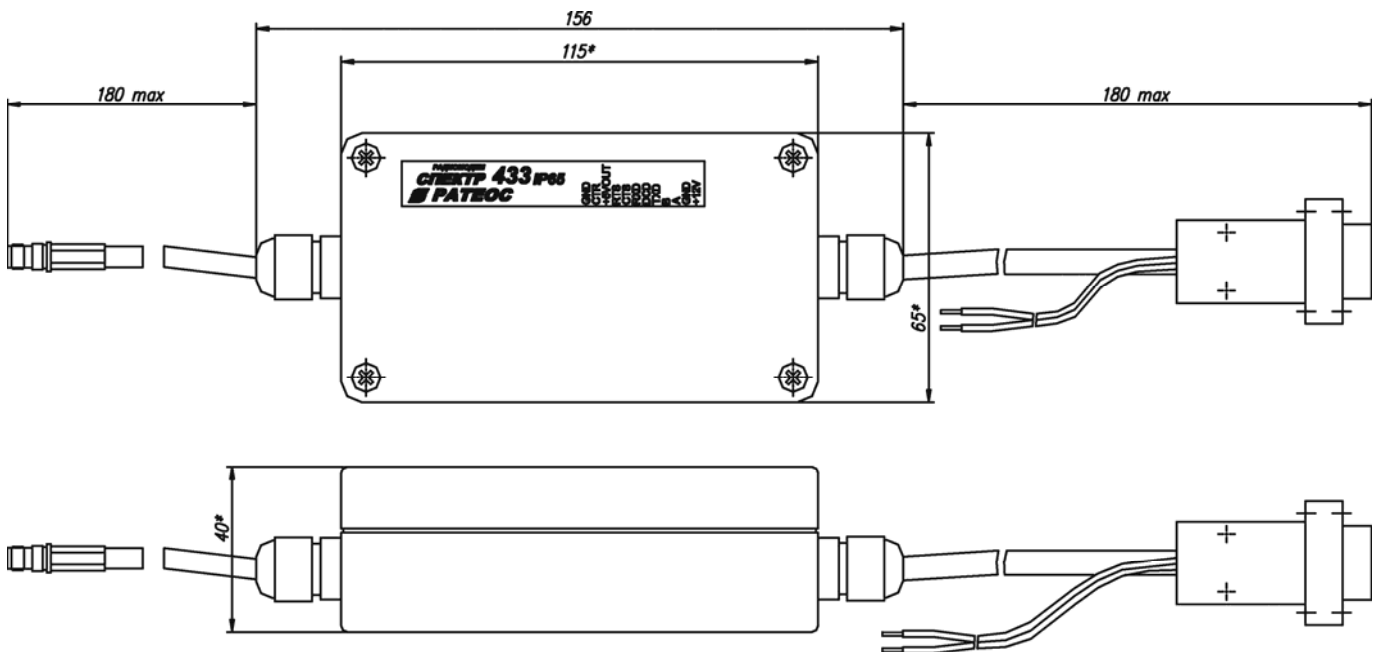
Исполнение IP65
