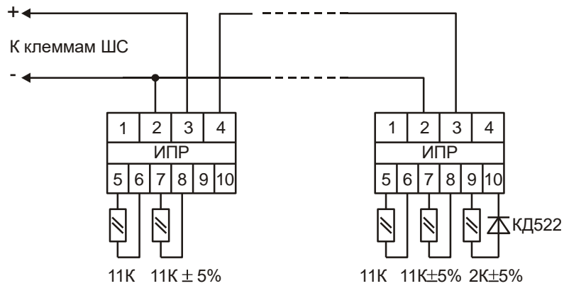
Рис. 8 Схема включения ручных ИП (ИПР и т. п.)
