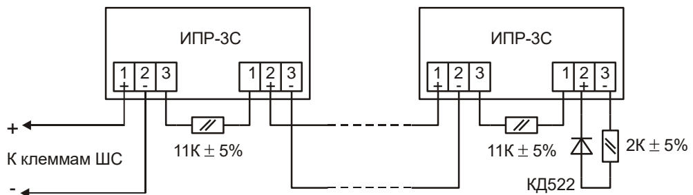
Рис. 13 Схема включения ИПР-3С
