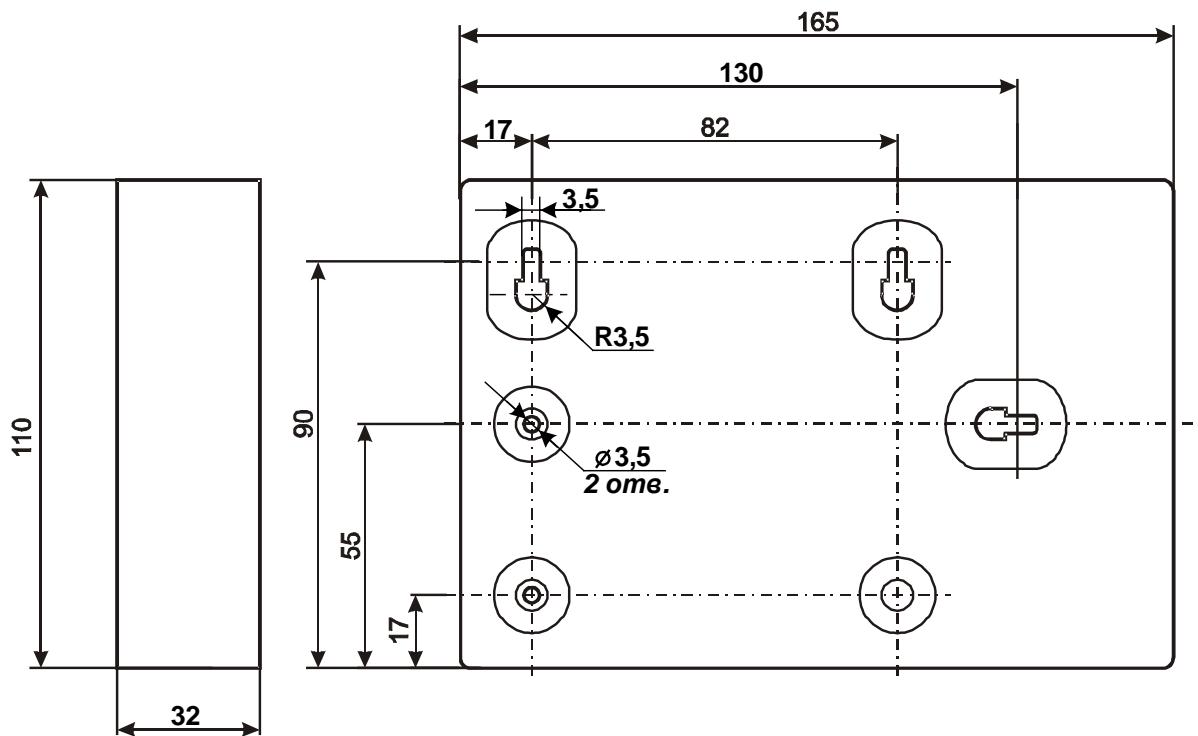
Рис. 4 Габаритные и присоединительные размеры (исполнение IP20)
