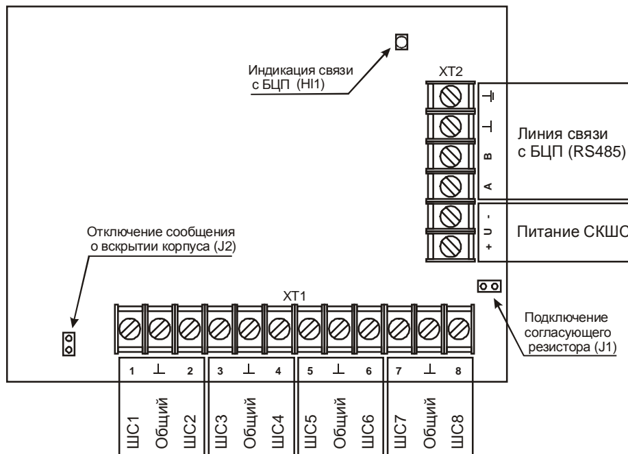
Рис. 6 Подключение СКШС
