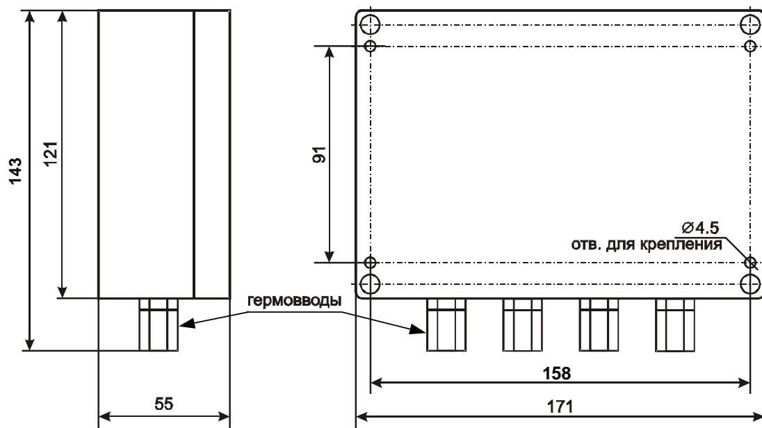
Рис. 3 Внешний вид, габаритные и присоединительные размеры (исполнение IP65)
