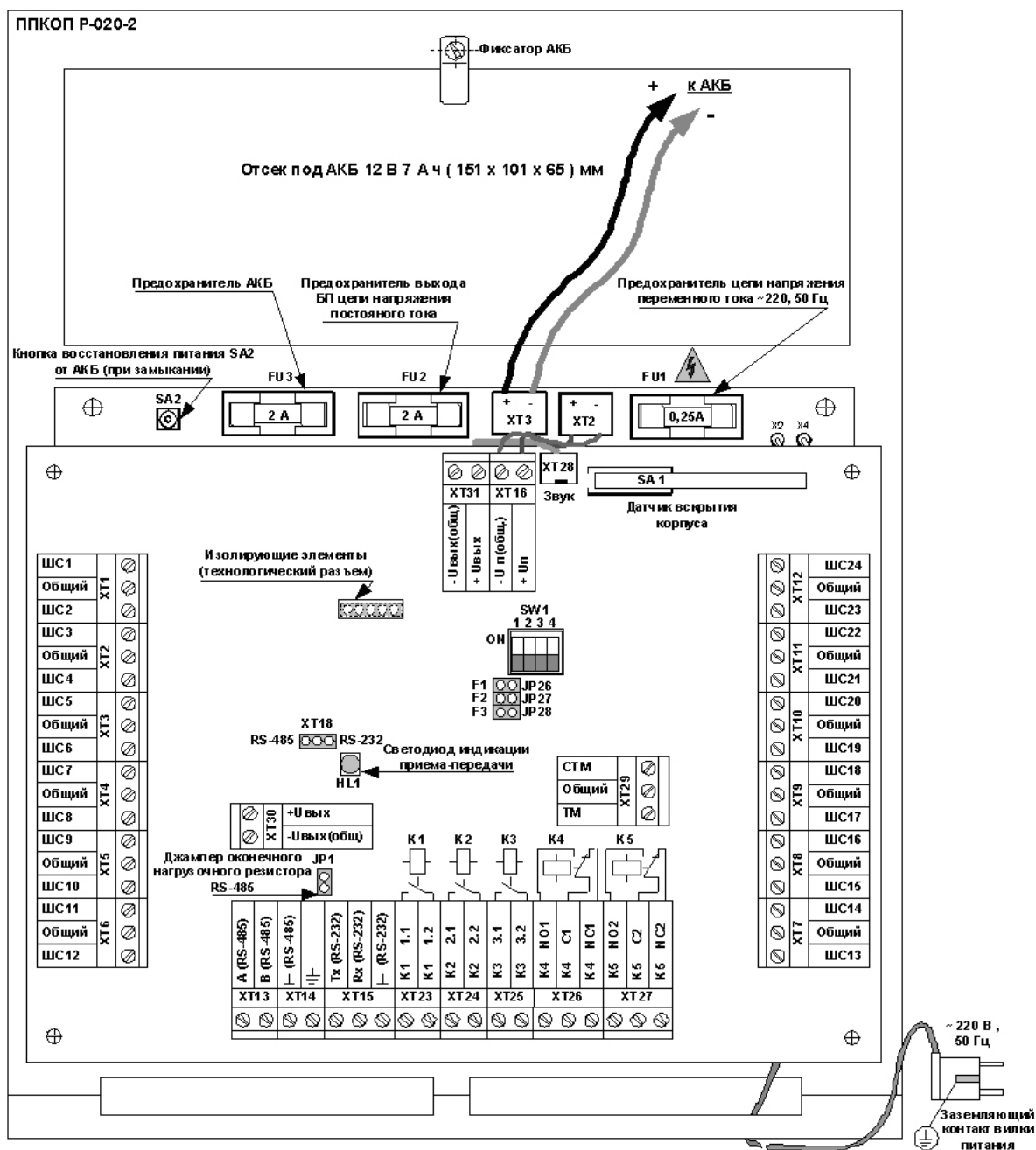
Рис. 17 Прибор исполнения Р-020-2 (с БП)
