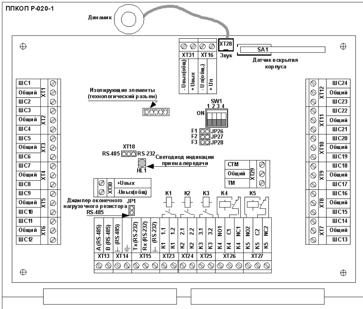
Рис. 16 Прибор исполнения Р-020-1 (без БП)
