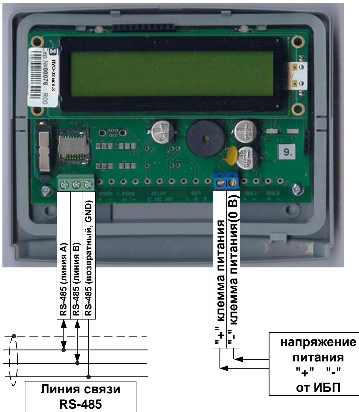
Рис. 7 Подключение ПУО
