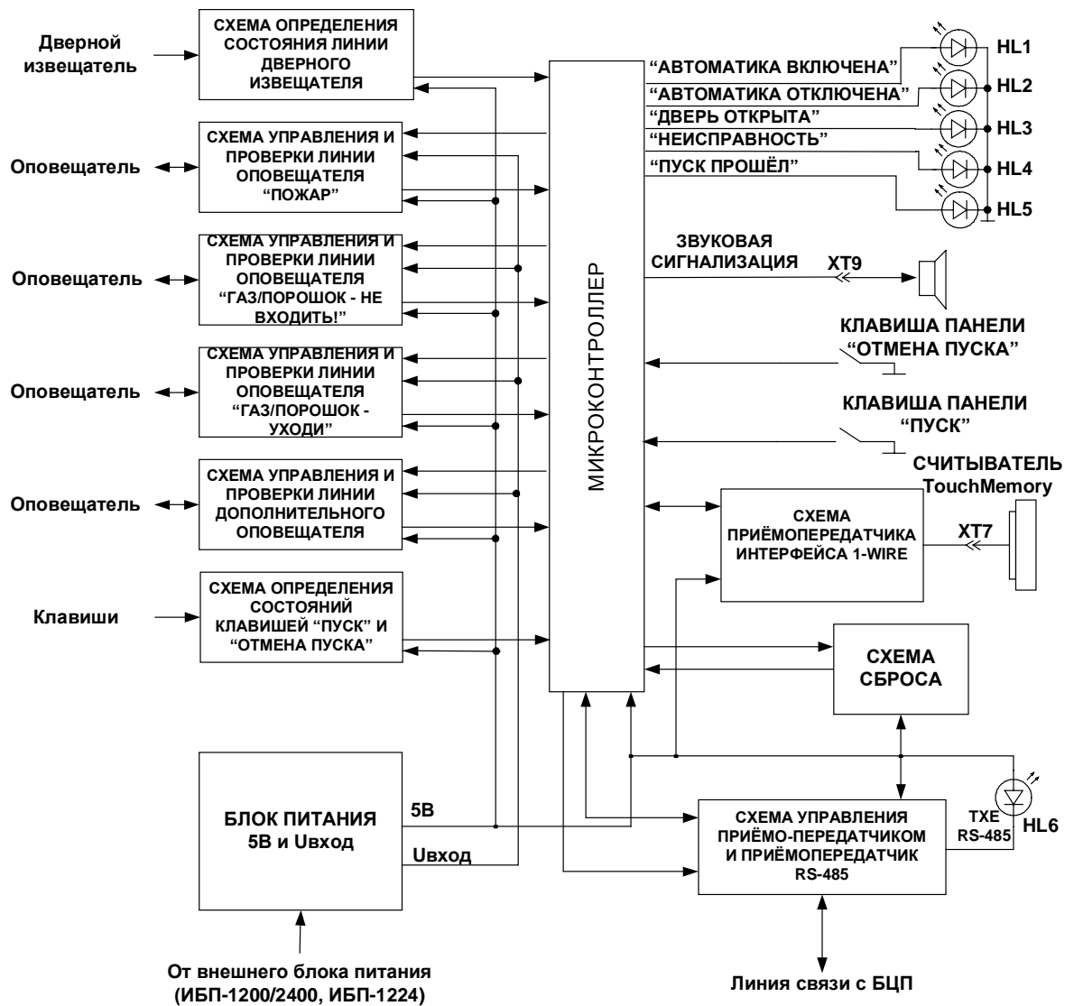
Рис. 3 Структурная блок-схема ППО
