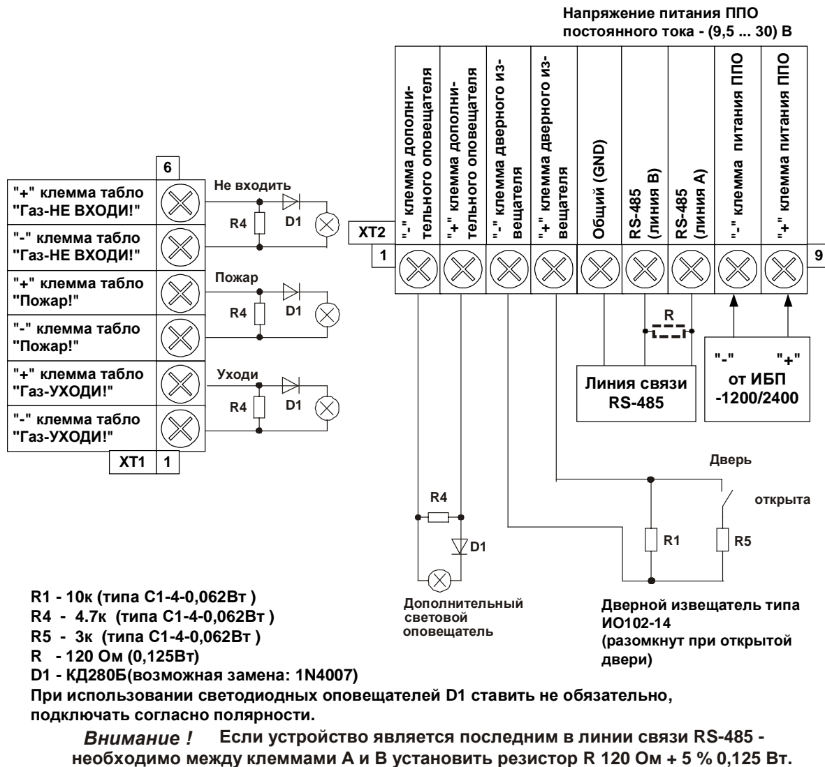
Рис. 5 Подключение ППО
