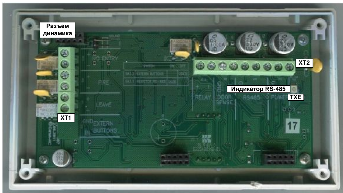
Рис. 2 Расположение элементов на плате ППО
