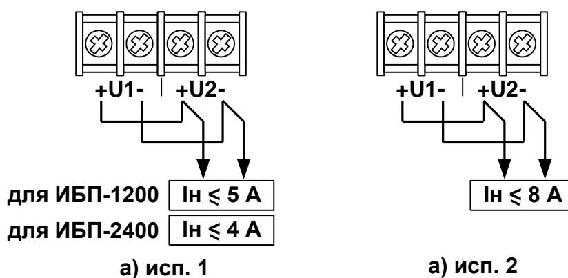
Рис. 6 Схема подключения нагрузки а) исп. 1 (для ИБП-1200 I_n \leq 5\text{A} ; для ИБП-2400 I_n \leq 4\text{A} ); б) исп. 2 ( I_n \leq 8\text{A} ).
