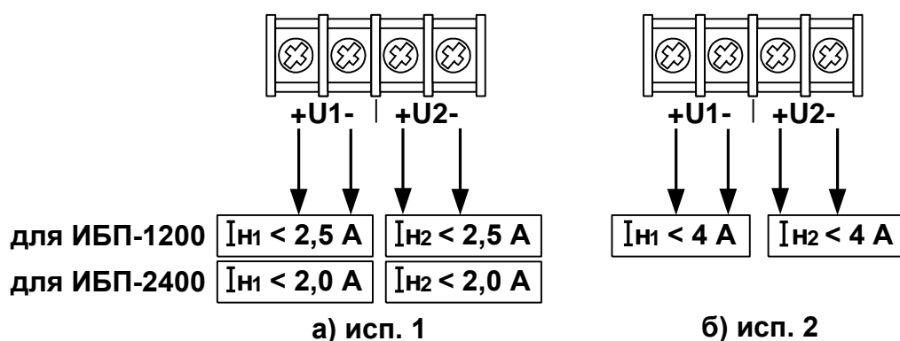
Рис. 5 Схема подключения нагрузки: а) исп. 1 (для ИБП-1200 I_{н1} < 2,5\text{A} ; I_{н2} < 2,5\text{A} ; для ИБП-2400 I_{н1} < 2,0\text{A} ; I_{н2} < 2,0\text{A} ); б) исп. 2 ( I_{н1} < 4\text{A} ; I_{н2} < 4\text{A} ).
