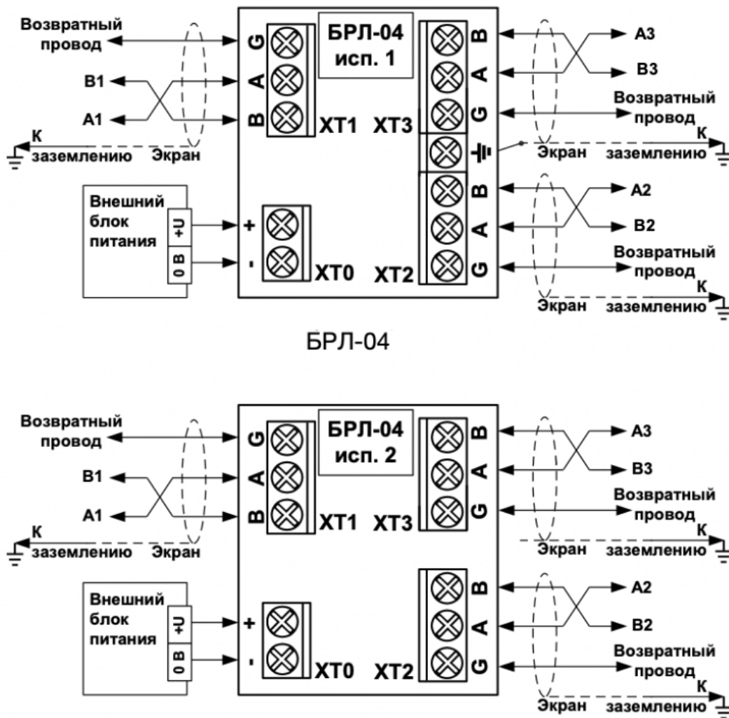
Рис. 4 Схема подключения БРЛ
