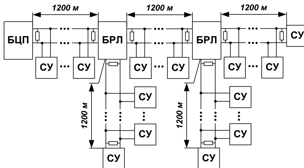
Рис. 5 Схема подключения БРЛ-04 для увеличения длины линии связи и гальванической развязки
