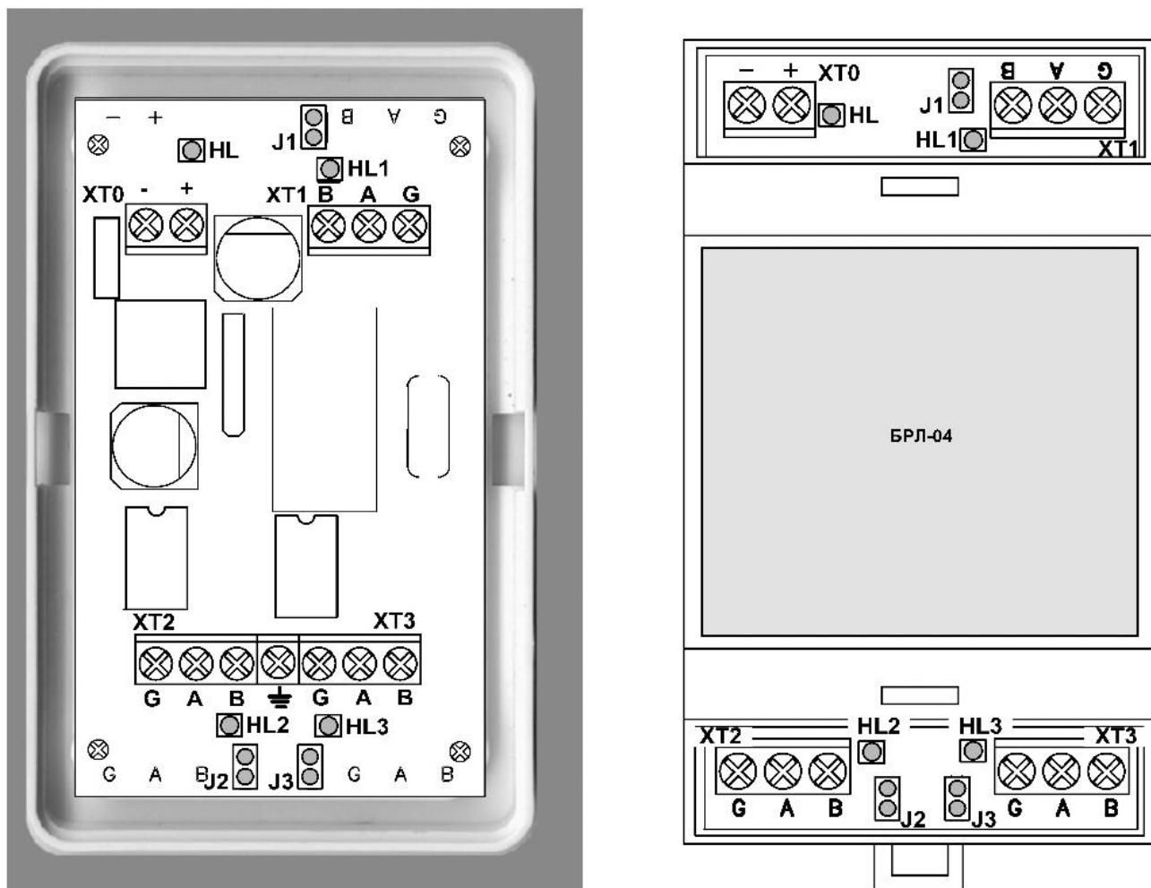
Рис. 2 БРЛ-04 и БРЛ-04 DIN. Расположение элементов.
