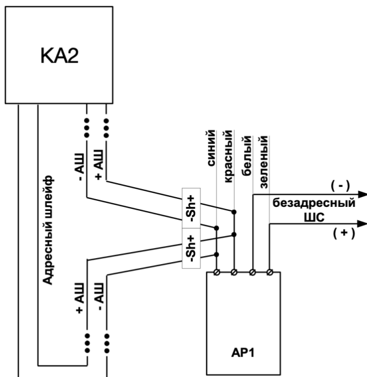
Рис. 2 Подключение AP1
