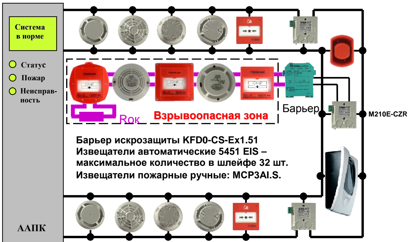
Рис.35. Схема подключения искробезопасных неадресных извещателей в адресно-аналоговый шлейф
