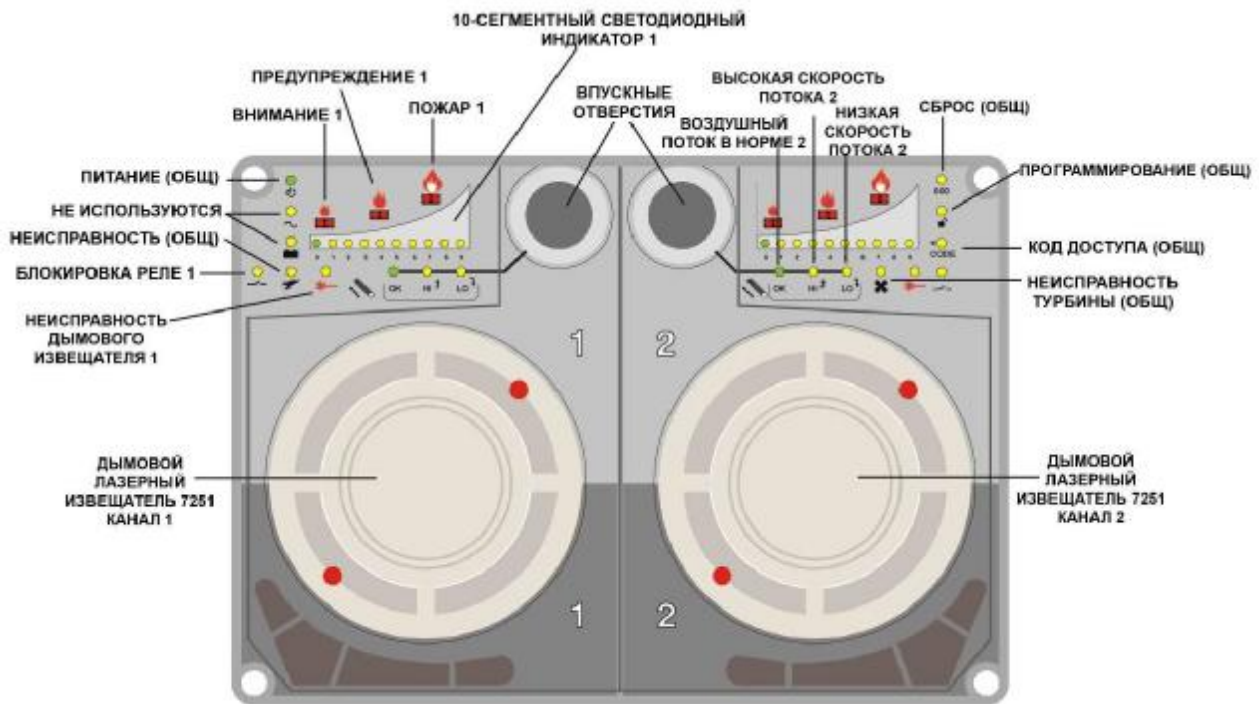
Рис. 27. Двухканальный извещатель LASD-2
