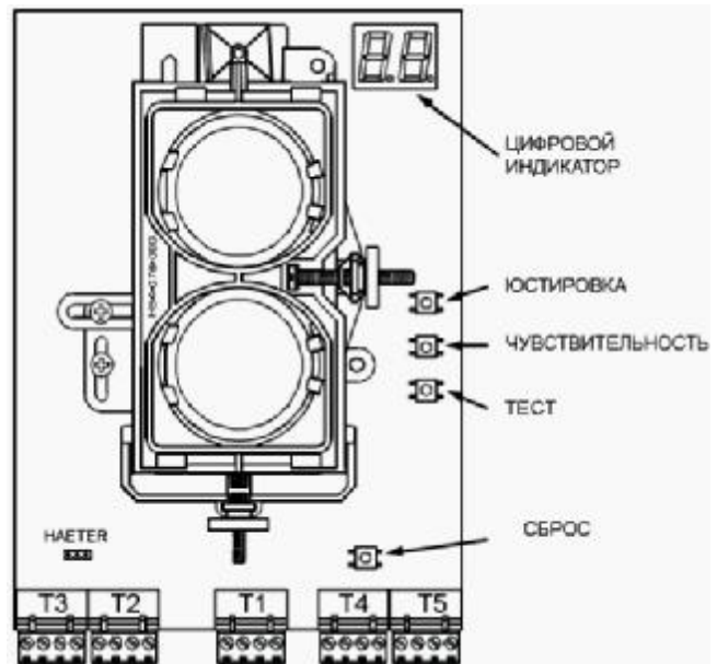
Рис. 20. Расположение цифрового индикатора, органов управления и терминалов
