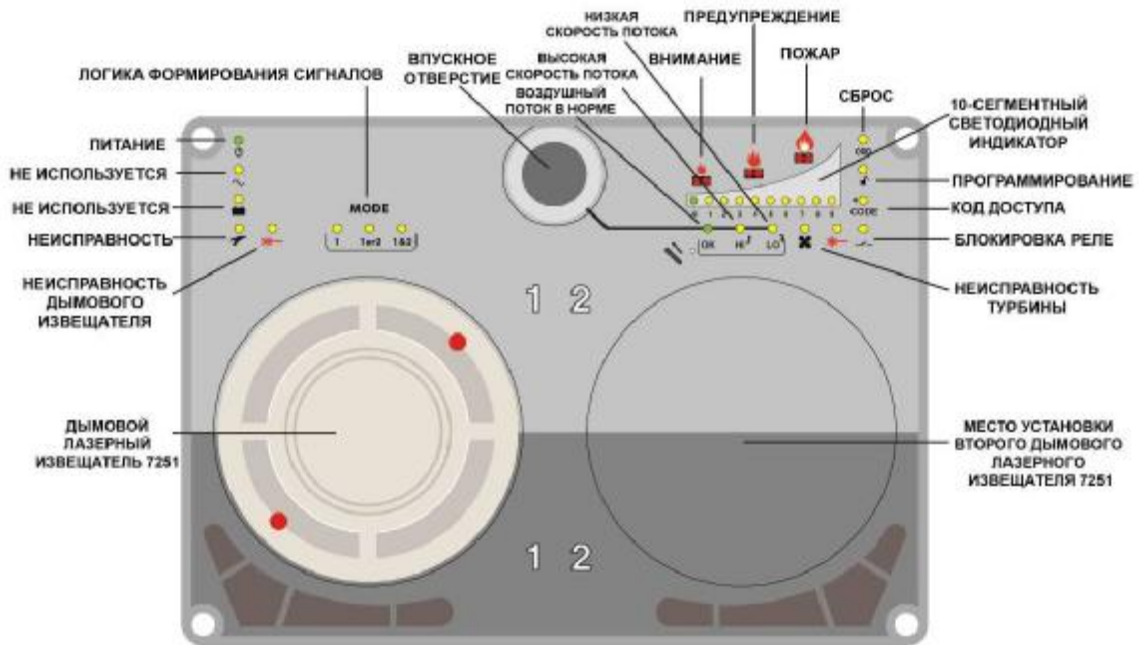
Рис. 26. Одноканальный извещатель LASD-1
